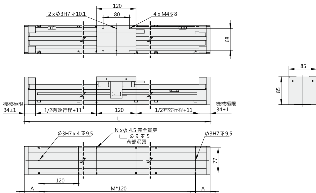
模組尺寸
