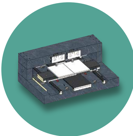
PCB板XRAY鑽通孔平臺
