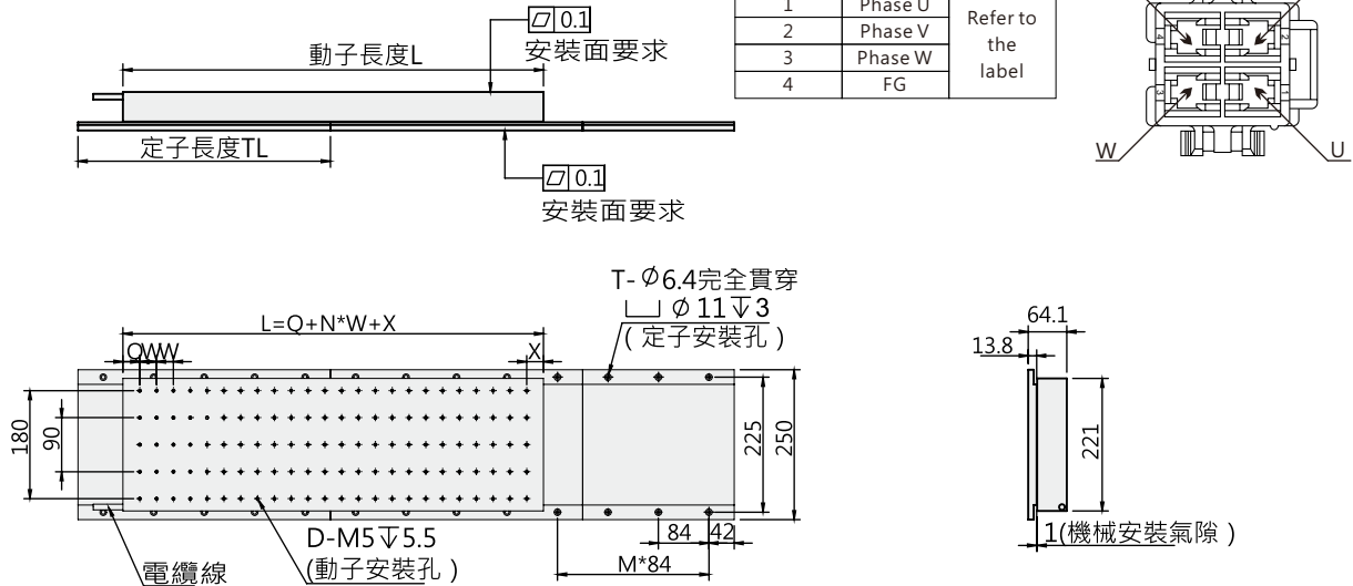
● 外形圖(單位:mm)
